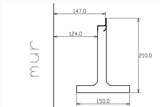
SA2 til gitterrist
